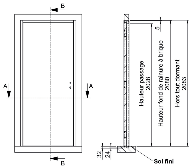
Coupe B-B
