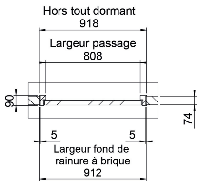
Coupe A-A
