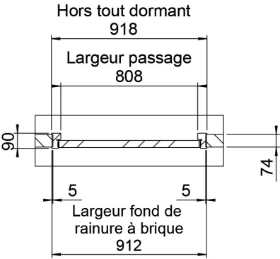
Coupe A-A
