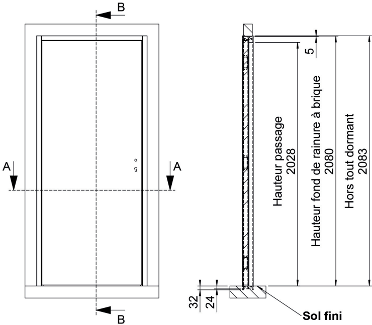
Coupe B-B
